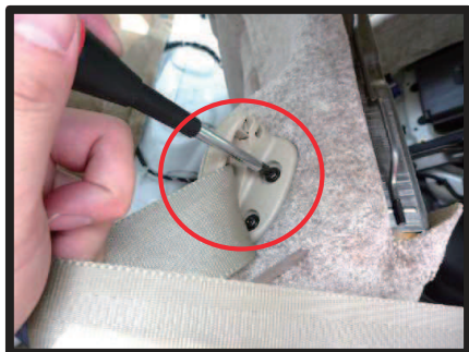
⑧背もたれ肩口のシートベルトガイドを+ドライバーを使用し、取り外します。（3箇所）
