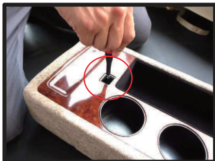
⑦ 図の赤丸部のネジを＋ドライバーを使用し外すと、プラスチックパーツが取り外せます。
