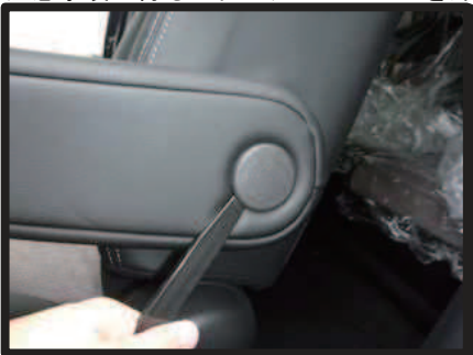
①ヘラ等を使用し、プラスチックを外します。
