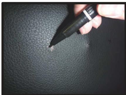
⑰4ページ⑥でパーソナルテーブルを取り外し、カバーを装着後、パーソナルテーブル取り付け位置にカバーの上から目印を付けます。(計6ヶ所)
