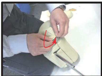
⑧ヘッドレストの内側へカバーを巻き込むようにします。
