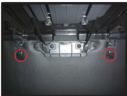
⑳取り外した逆の手順で、パーソナルテーブルを元に戻します。 ⑲で開けた穴は、○部分の裏にある突起物の固定に必要な穴です。
