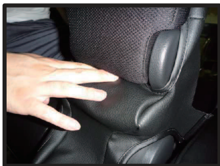
⑨アームレスト下側に生地を入れ込みます。
