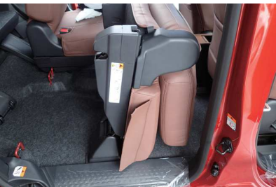
2 列目シートタンブル状態
