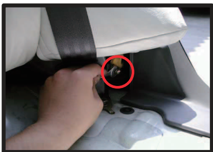
⑰ネジを取付けシートを固定します。
